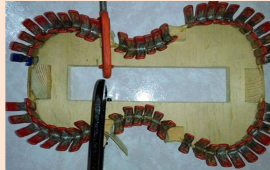
圖 10: 背板黏好後拆掉內模
