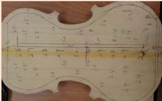
圖 8: 面板厚度數據
